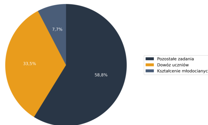
Ryc. 10.5.3. Wydatki na zadania specjalne
